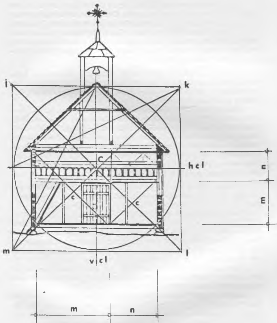
BRĖŽINYS 2: SKERSINIS PIŪVIS
