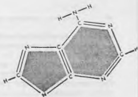
Adeninas
