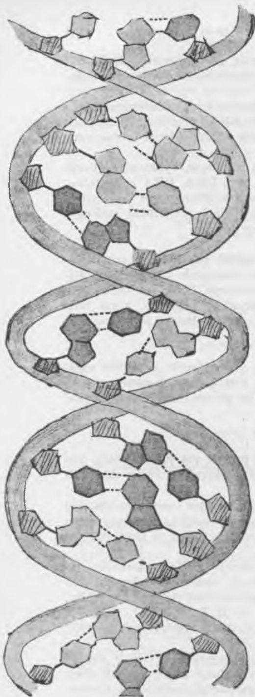
Pav. 6. Deoksiribonuklejinė rūgštis. Spiralinė yra deoksiribozės ir fosforo rūgšties polimerai. Taškų linijos — vandenilio ryšiai tarp bazių
