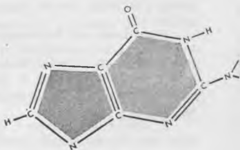
Gvaninas
