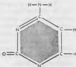
Citozinas
