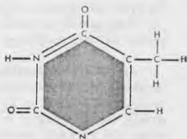
Timinas
