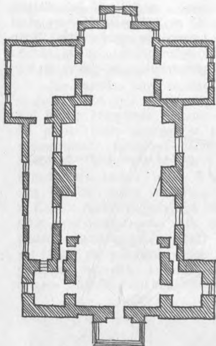
13 pav. Benediktinių vienuolyno bažnyčios sche- ma, sudaryta pagal 1893 m. inventorizacijos brėžinį
