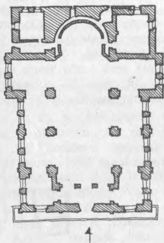
6 pav. Jėzuitų vienuolyno bažnyčios plano schema, sudaryta pagal 1823m. brėžinį
