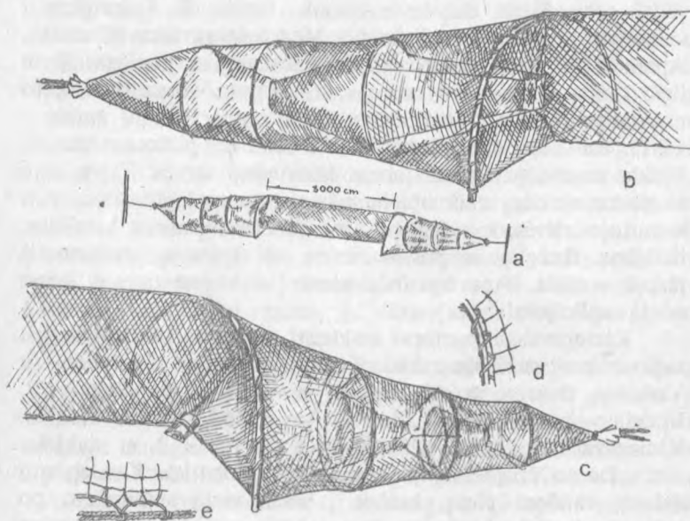
2 pav. Venteris, Kražių ap., Paežerio k.: a - bendras vaizdas, b, c - venterio galai, d - tinklo tvirtinimas prie medinio lanko, e - tinklo tvirtinimas prie lanko galus jungiančios virvelės
