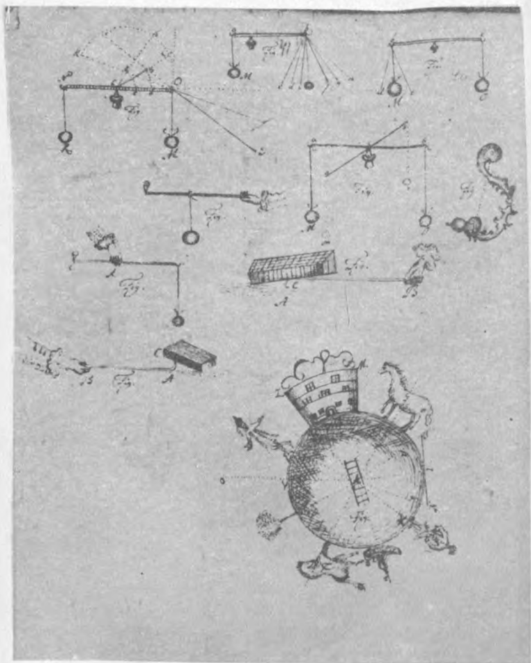
8a ir 8b pav. Brėžiniai, iliustruojantys I. Lappos mechanikos kursą
