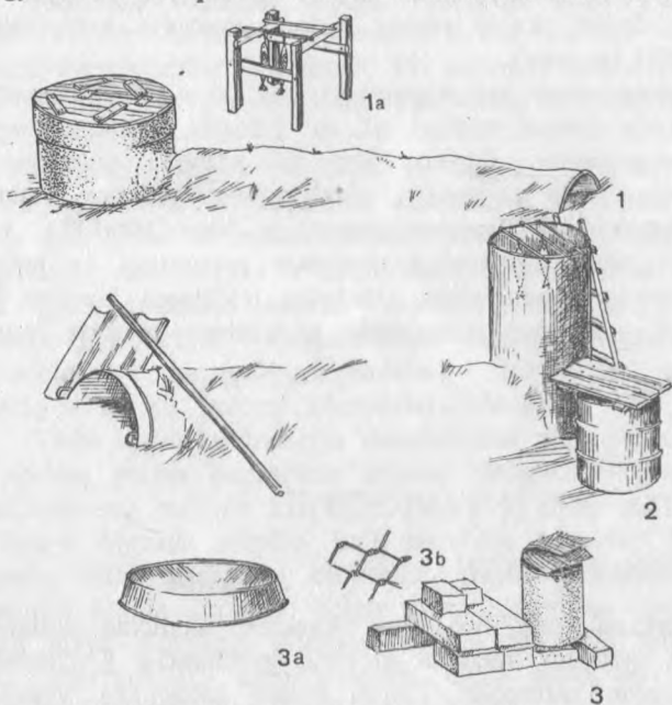
9 pav. Rūkyklos. Sakalausų, Kražių ap., Vaitkiškių k.: 1 - bendras vaizdas, 1a - medinis rėmas žuvims kabinti; 2 - P. Vedeikio, Pupėnų k., V. Butkevičiaus, Paežerio k.; 3 - bendras vaizdas, 3a - skardinė vonelė, užvožiama ant rūkyklos viršaus, 3b - metalinis tinklėlis
