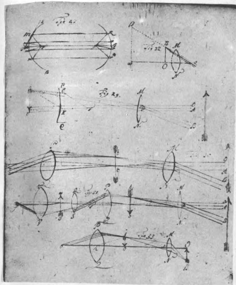
6a ir 6b pav. Brėžiniai, iliustruojantys optikos reiškinius, regos fenomeną, vaizdų susidarymą optinėse sistemose
