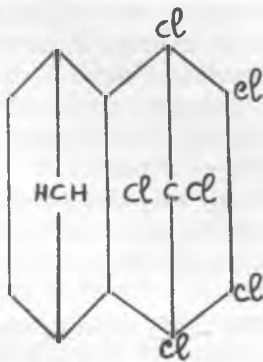
Aldrinas
