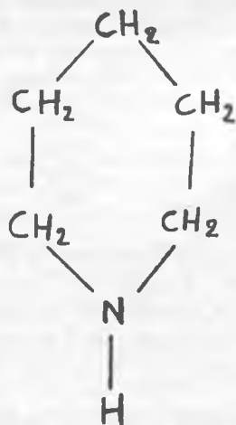
Piperidinas
