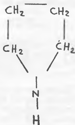
Pirolidinas
